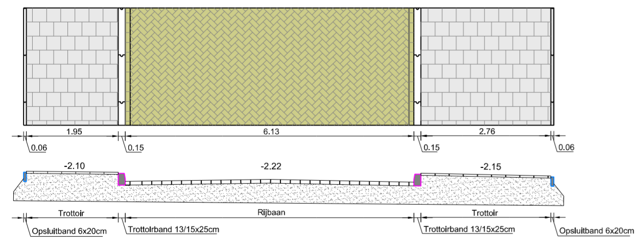
bestaand dwarsprofiel
