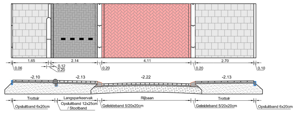
nieuw dwarsprofiel
