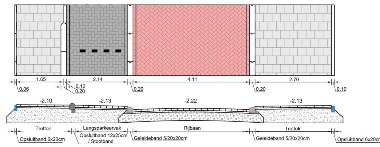
nieuw dwarsprofiel
