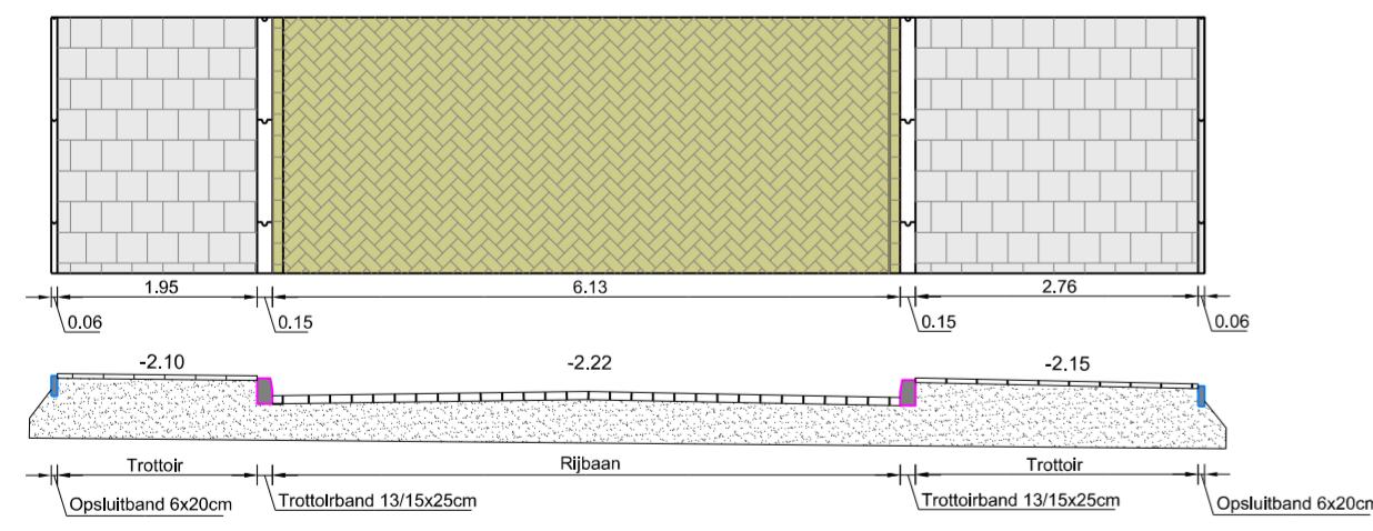
bestaand dwarsprofiel
